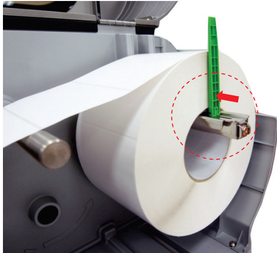
3 吋标签供应轴
